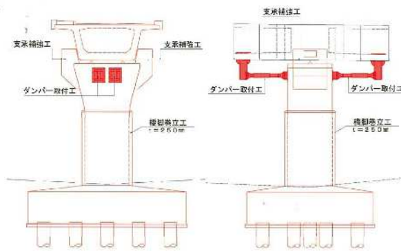
ダンパー設置図(正面図)
