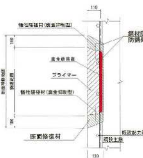
断面修復工（完了）
