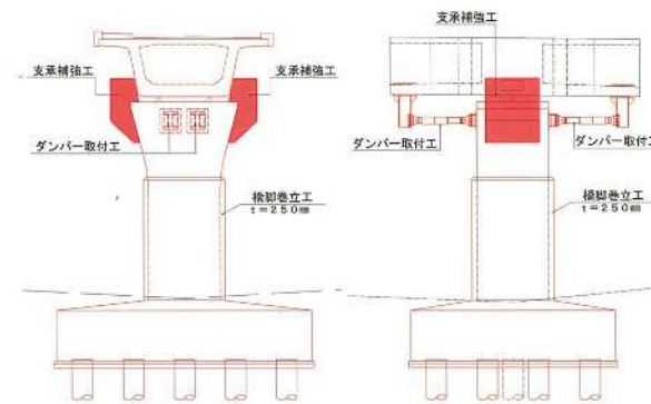
支保補強工施工図(正面図)
