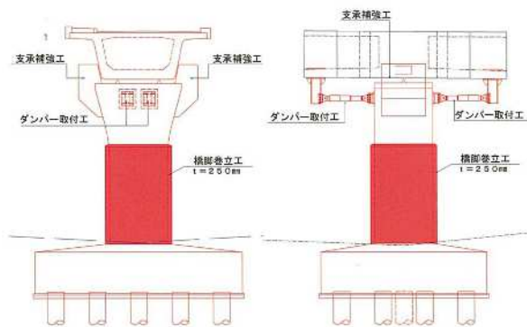
橋脚巻立工図(正面図)
